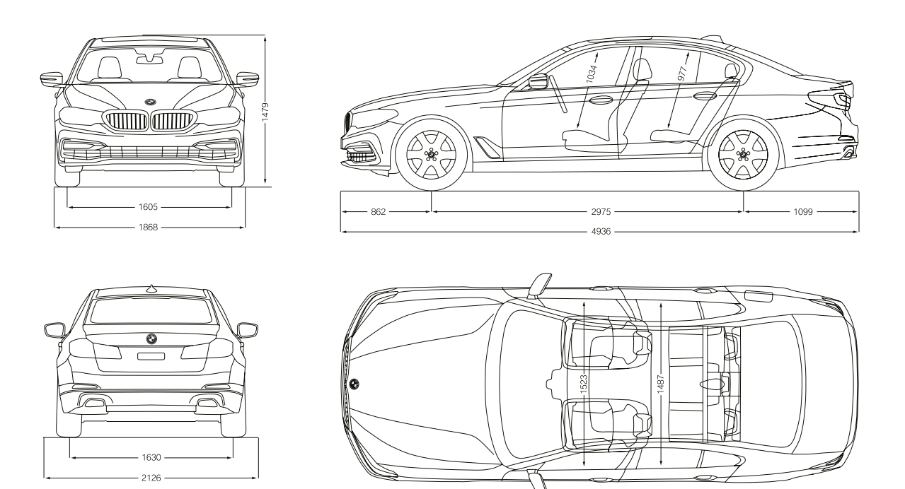
Alle Maßangaben der technischen Zeichnung in Millimeter. Höhe ohne Dachantenne beträgt 1466 mm. Angaben zu Fahrleistung, Verbrauch und CO 2 -Emission gelten für Fahrzeuge mit Seriengeräte.
