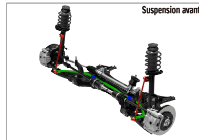
Suspension avant
