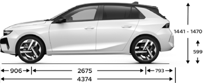
Astra 5 portes Toutes les dimensions en mm
