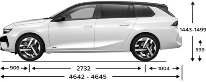
Astra Sports Tourer Toutes les dimensions en mm
